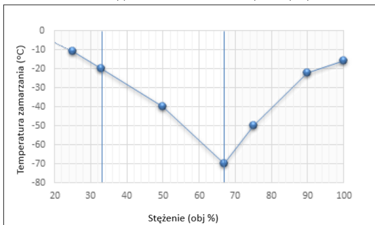
Schemat zależności ochrony przed zamarzaniem mieszaniny Kemetyl Płynu do chłodziw GlycoCool Premium 774 C z wodą
