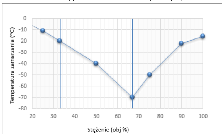
Schemat zależności ochrony przed zamarzaniem mieszaniny Kemetyl Płynu do chłodziw GlycoCool Longlife Premium 774 D-F z wodą
