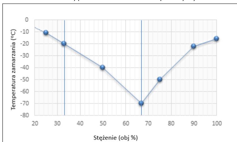
Schemat zależności ochrony przed zamarzaniem mieszanki Kemetyl Płynu do chłodziw GlycoCool Premium Longlife 774 D-F z wodą
